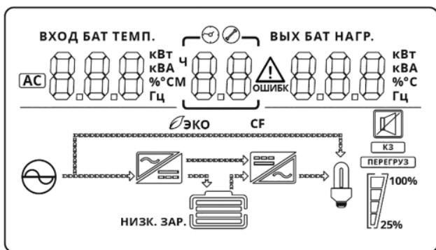
Рисунок 4.2. ЖК-дисплей
