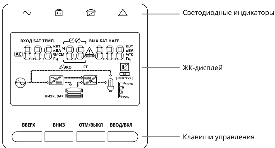
Рисунок 4.1. Панель управления ИБП
