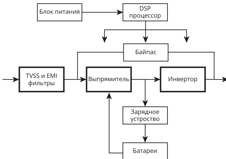
Рисунок 2.5. Система ИБП
